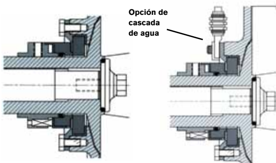
Tipo 1: Sello equilibrado externo con superficie de contacto reemplazable Tipo 1: Con opción de cascada de agua
